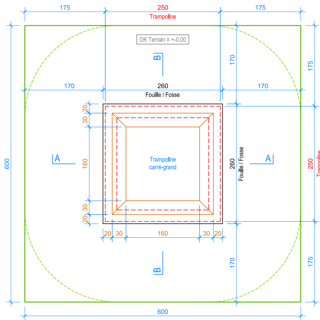
PLAN 1:50
