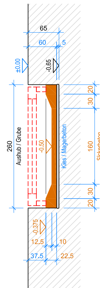
SCHNITT B-B 1:50
