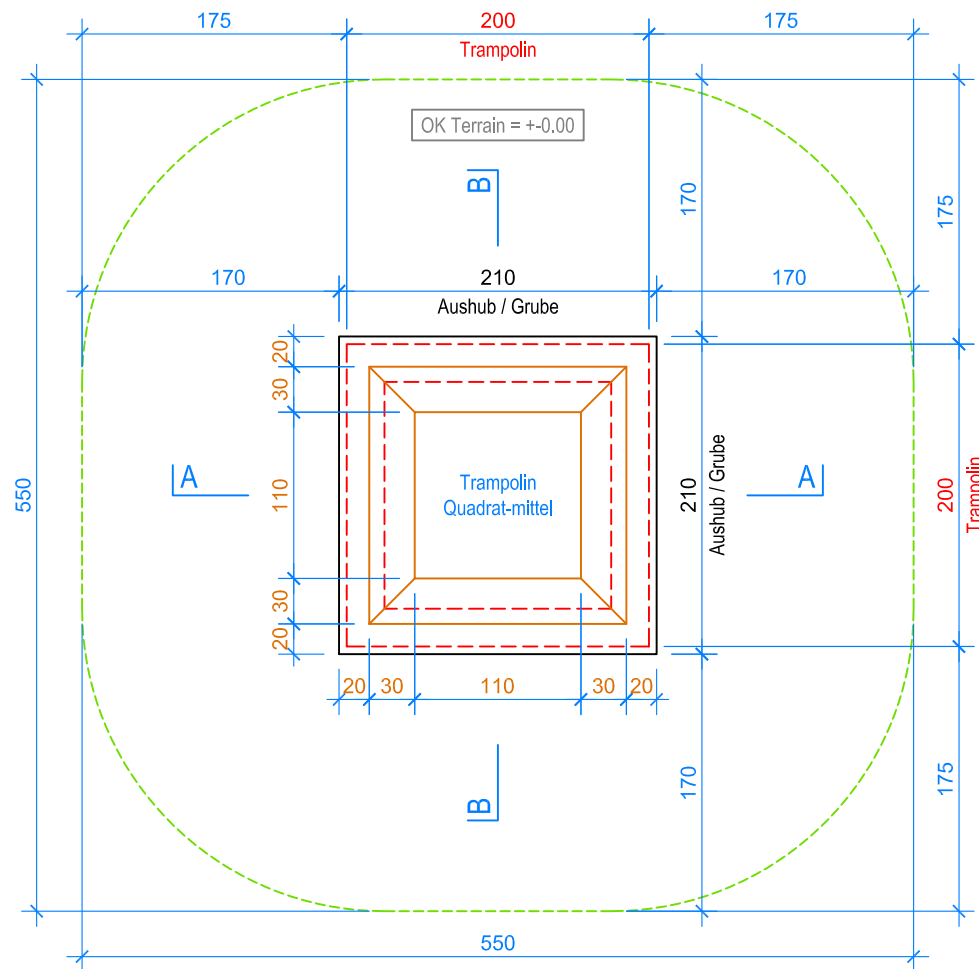
GRUNDRISS 1:50
