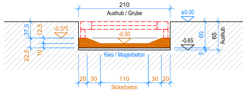
SCHNITT A-A 1:50
