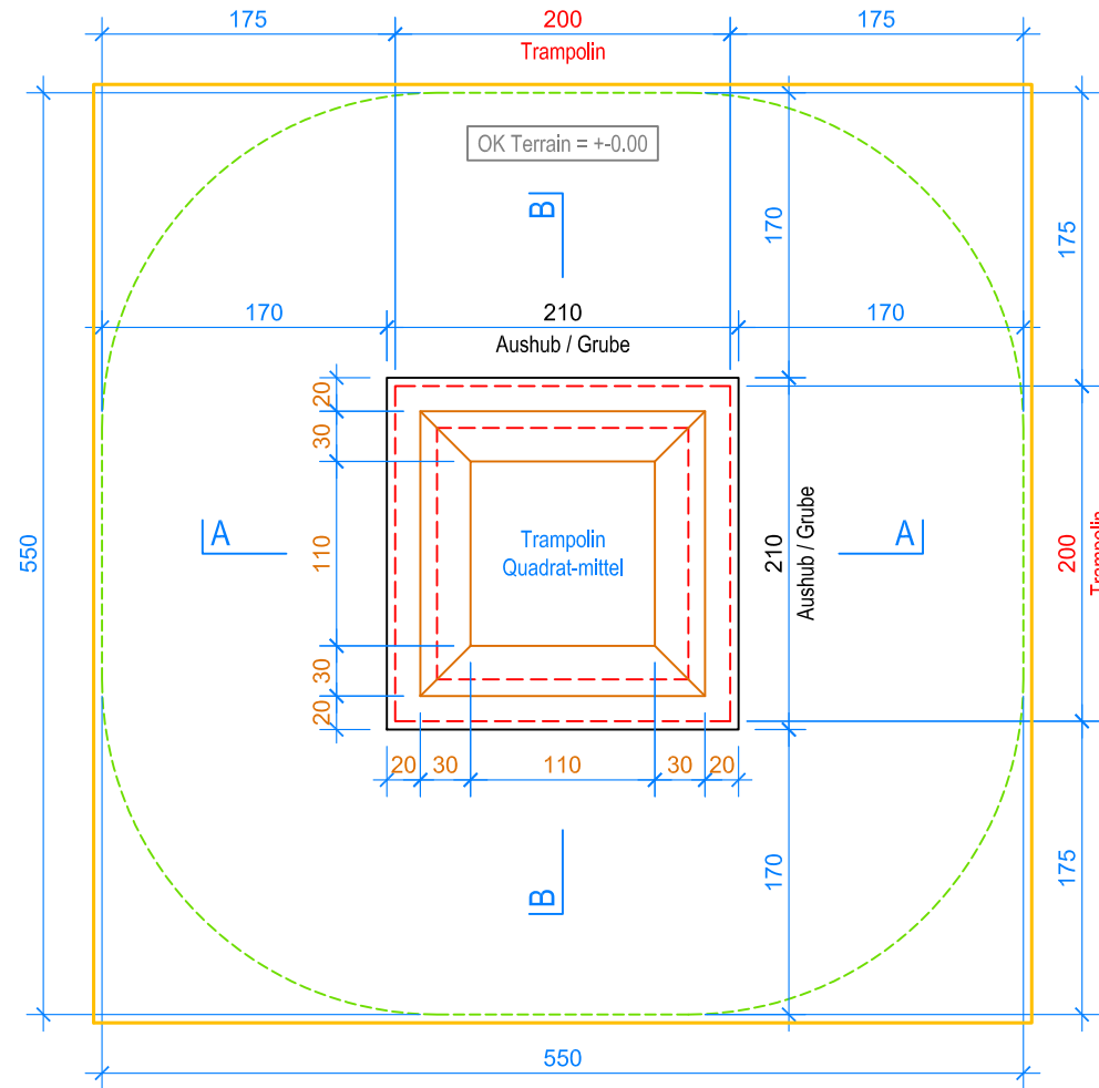
GRUNDRISS 1:50
