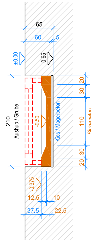
SCHNITT B-B 1:50
