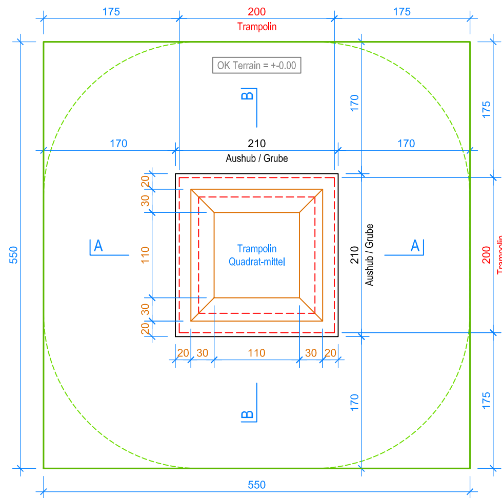
GRUNDRISS 1:50
