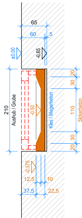
SCHNITT B-B 1:50
