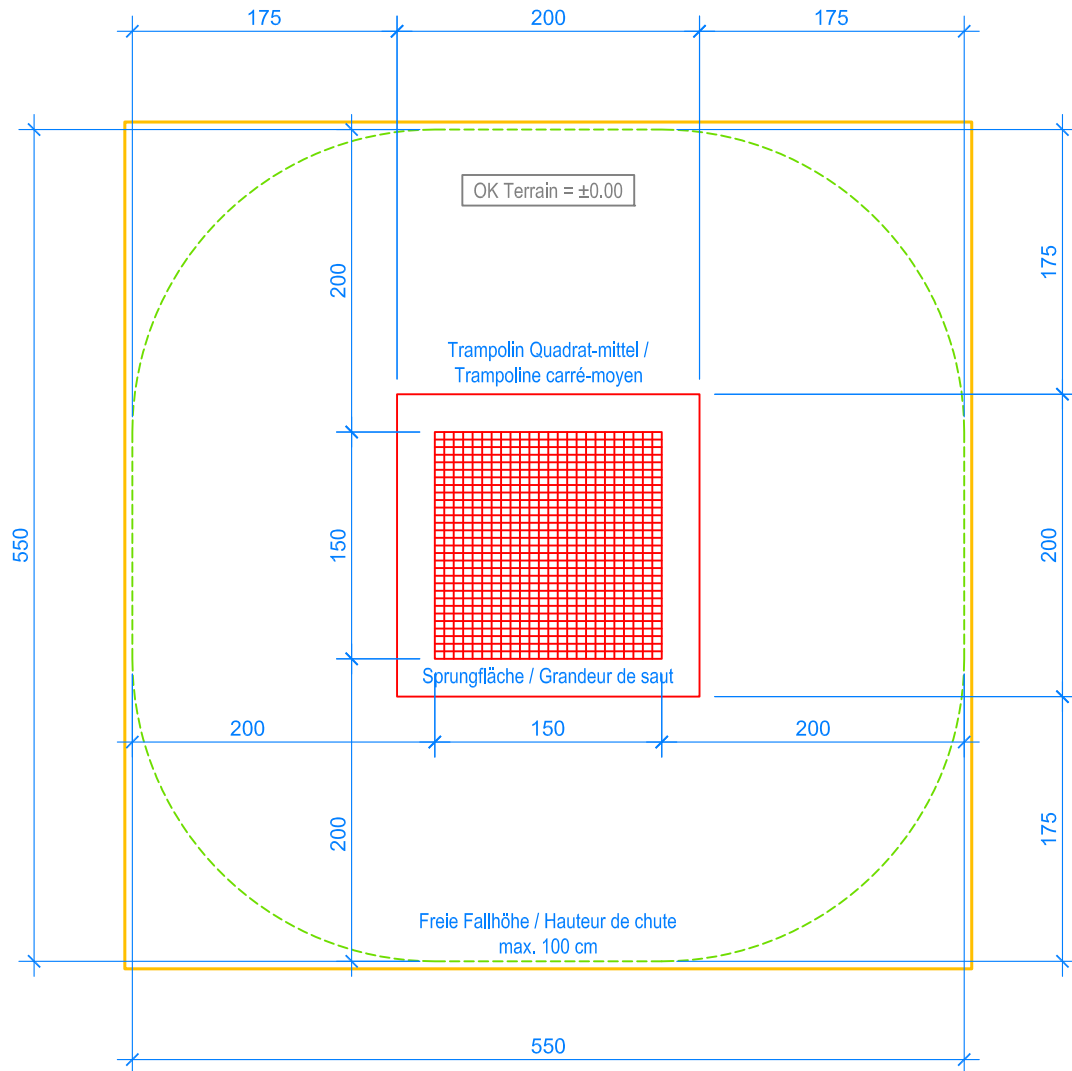
GRUNDRISS / PLAN 1:50
