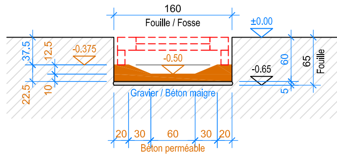
COUPE A-A 1:50
