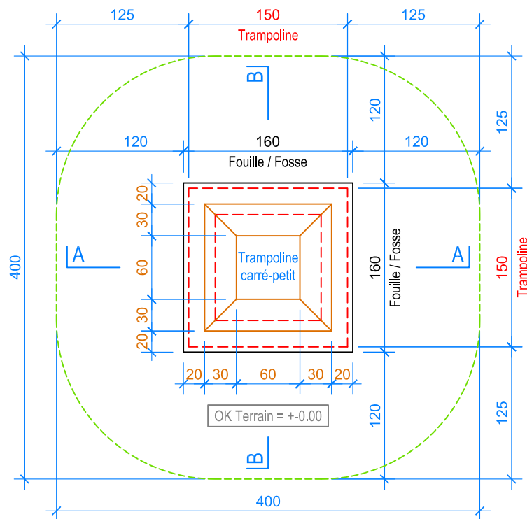
PLAN 1:50
