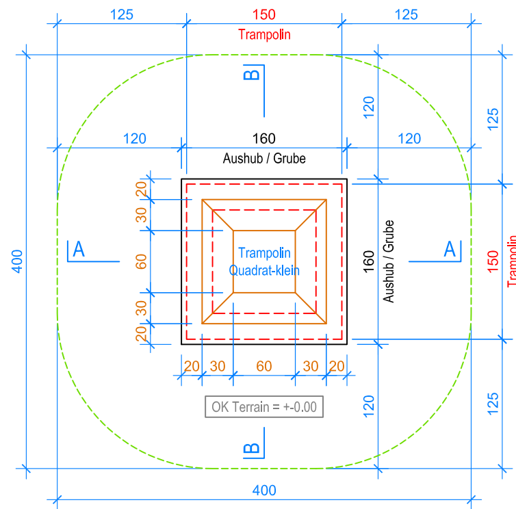
GRUNDRISS 1:50
