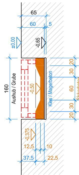
SCHNITT B-B 1:50
