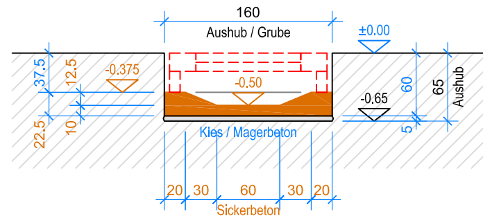
SCHNITT A-A 1:50
