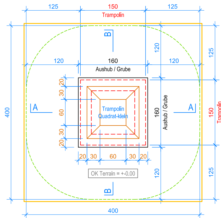
GRUNDRISS 1:50
