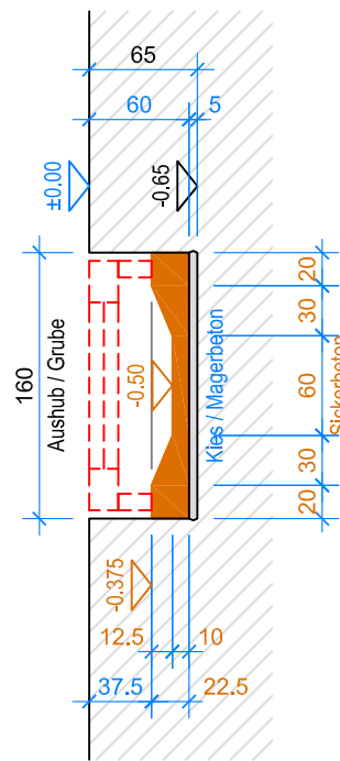
SCHNITT B-B 1:50
