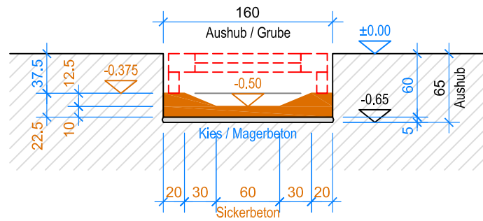
SCHNITT A-A 1:50
