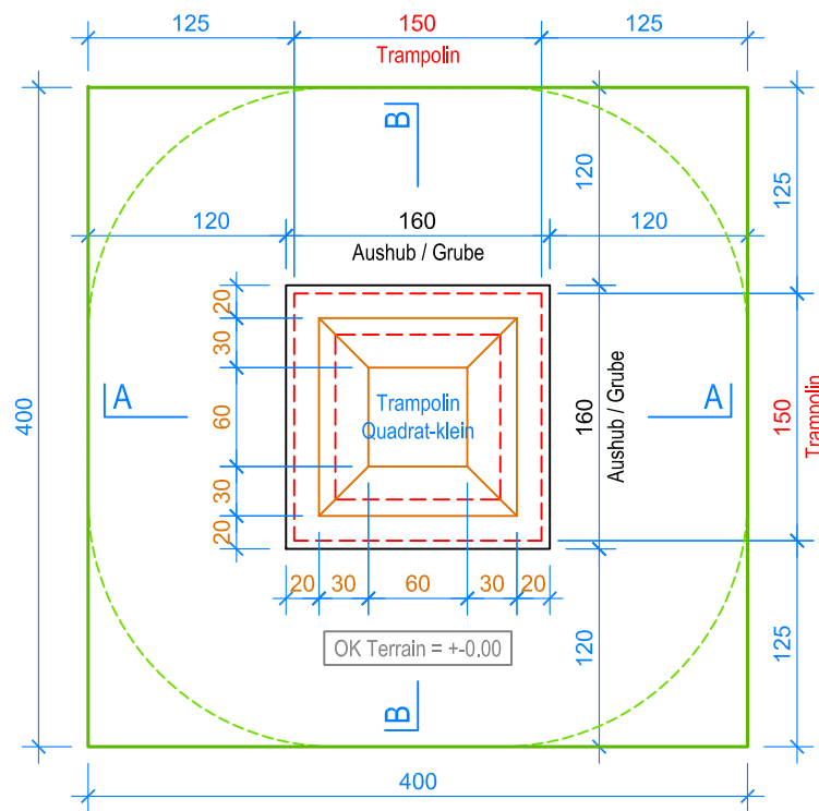
GRUNDRISS 1:50
