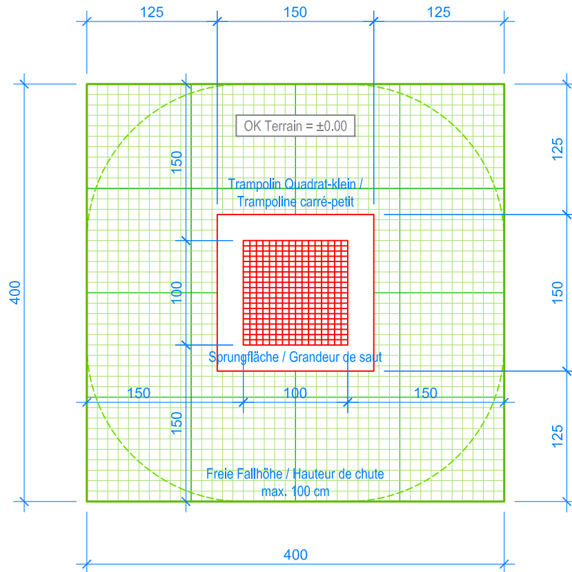
GRUNDRISS / PLAN 1:50
