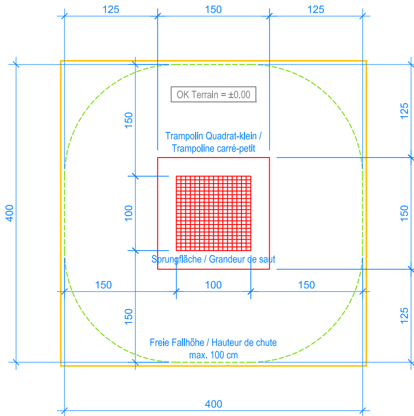
GRUNDRISS / PLAN 1:50
