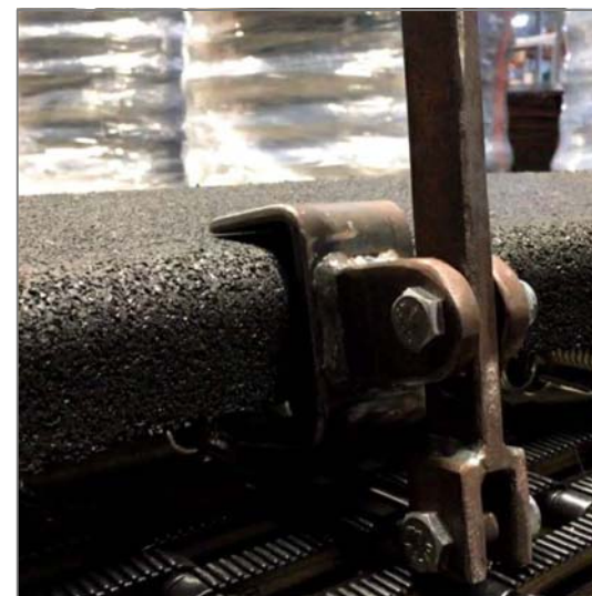
Photo-3 : Débander le ressort avec l'outil à crochet
