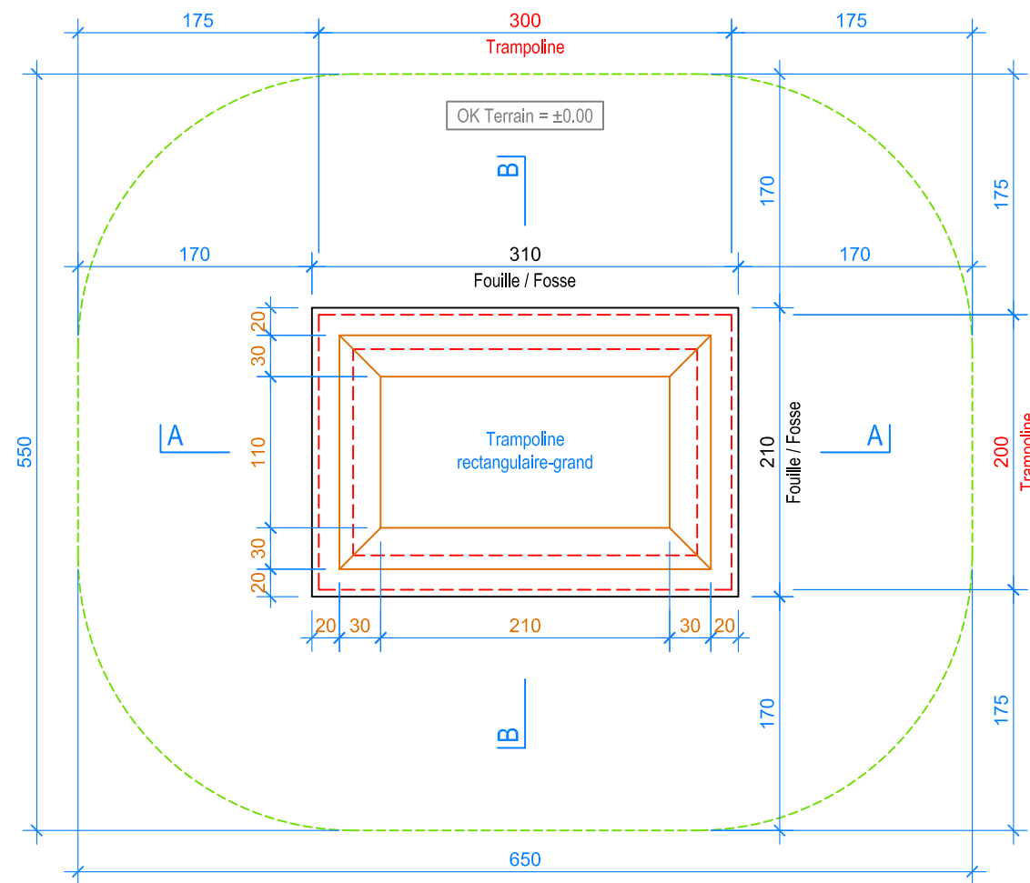
PLAN 1:50
