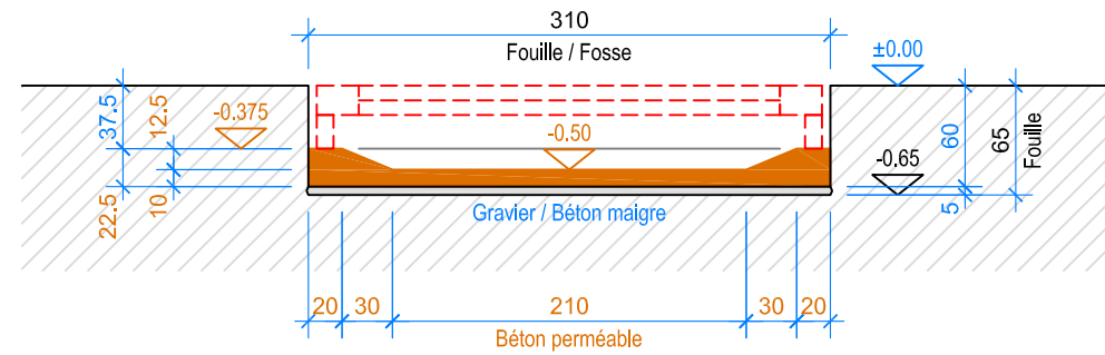
COUPE A-A 1:50
