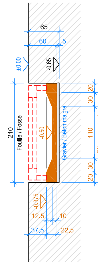
COUPE B-B 1:50
