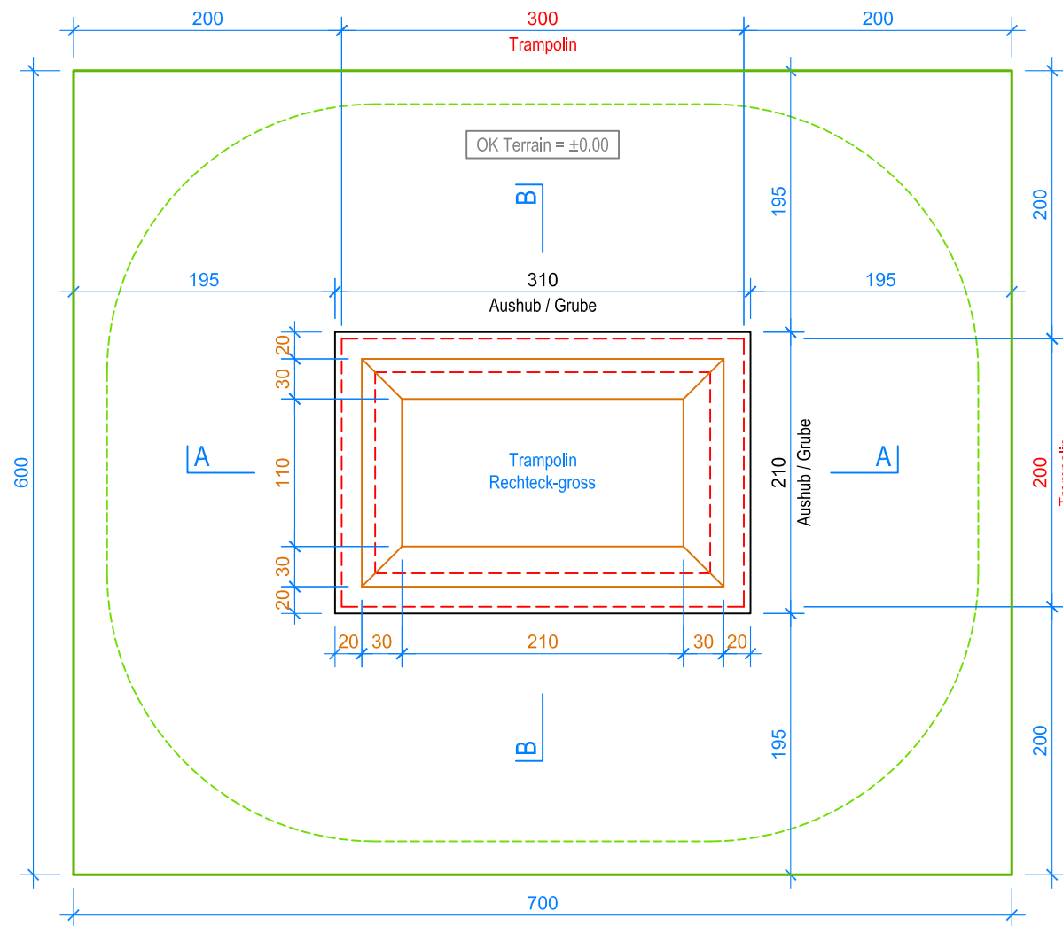
GRUNDRISS 1:50
