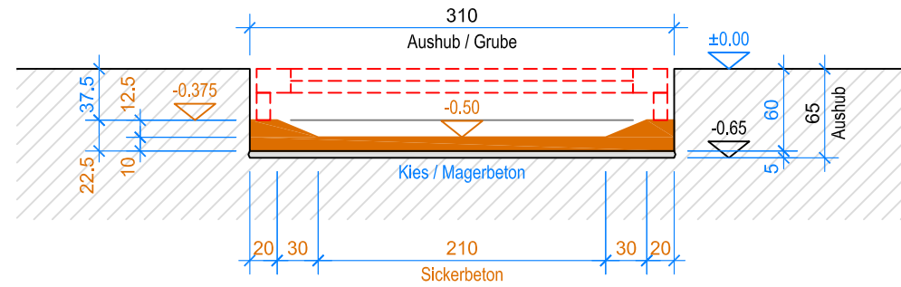
SCHNITT A-A 1:50
