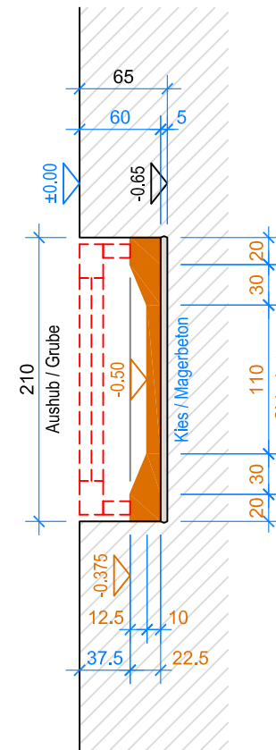
SCHNITT B-B 1:50
