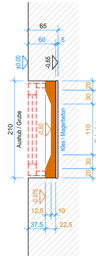
SCHNITT B-B 1:50
