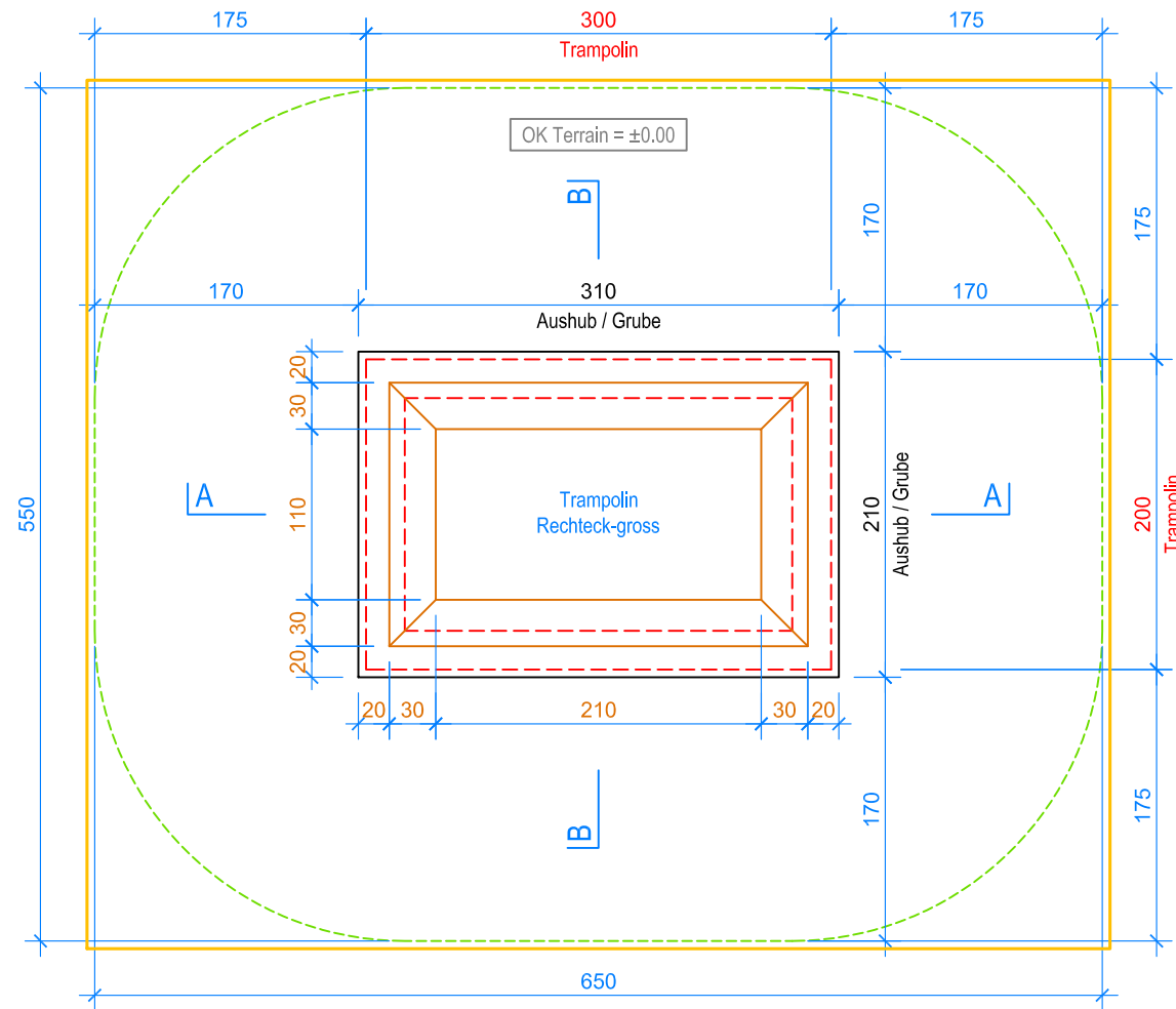
GRUNDRISS 1:50
