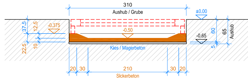
SCHNITT A-A 1:50
