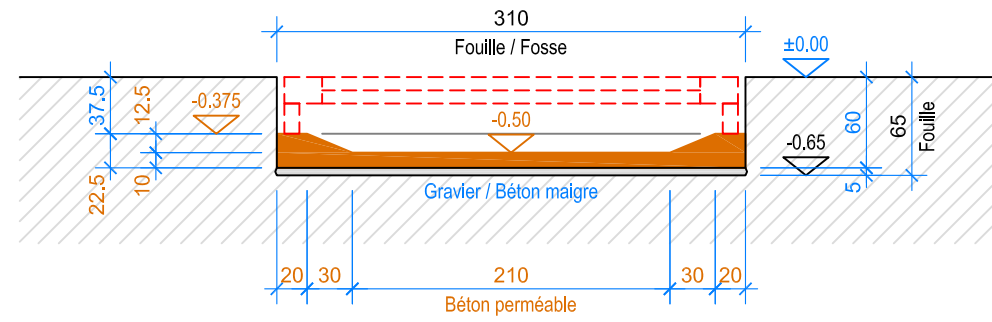
COUPE A-A 1:50
