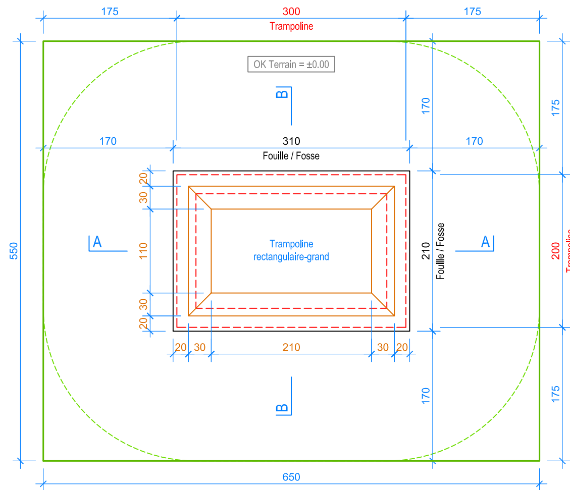
PLAN 1:50
