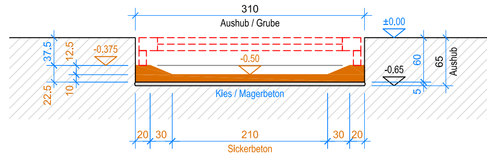
SCHNITT A-A 1:50
