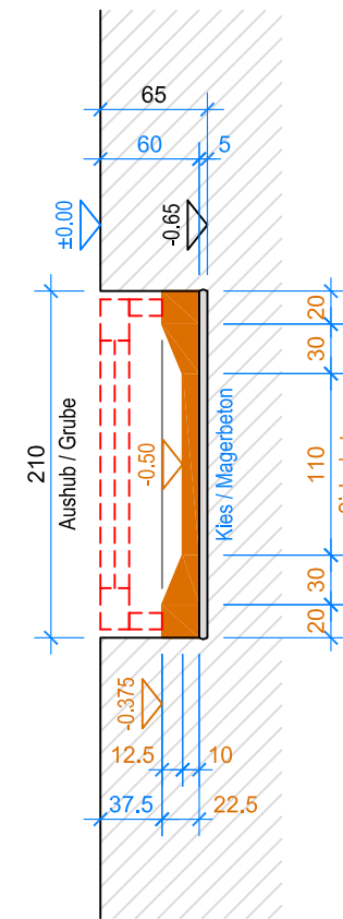
SCHNITT B-B 1:50
