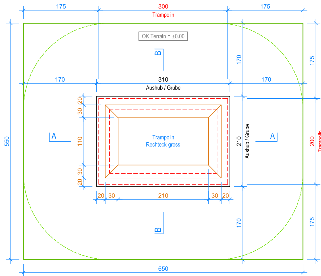
GRUNDRISS 1:50
