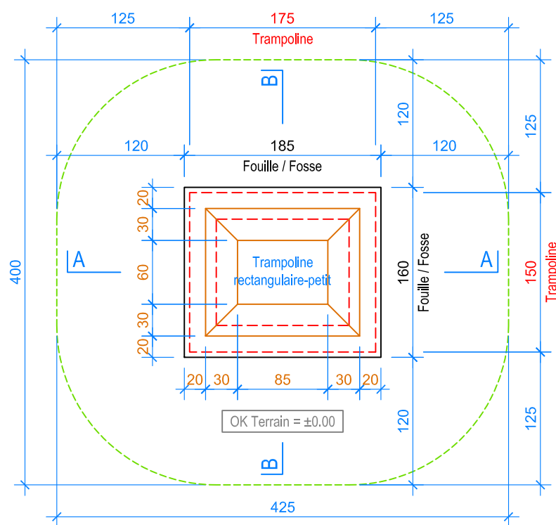
PLAN 1:50
