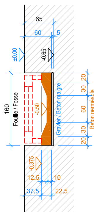
COUPE B-B 1:50
