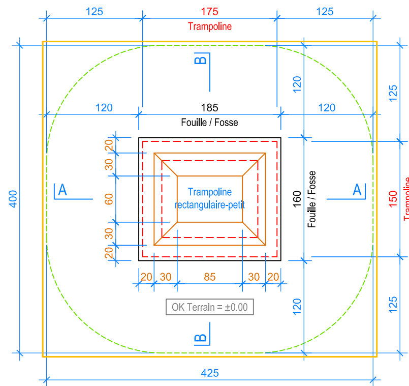
PLAN 1:50
