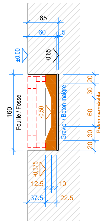
COUPE B-B 1:50
