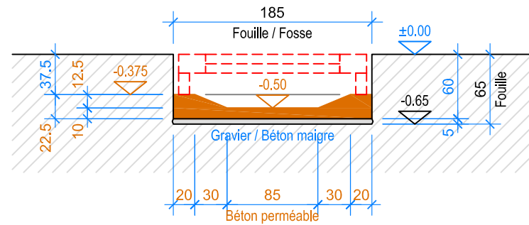
COUPE A-A 1:50
