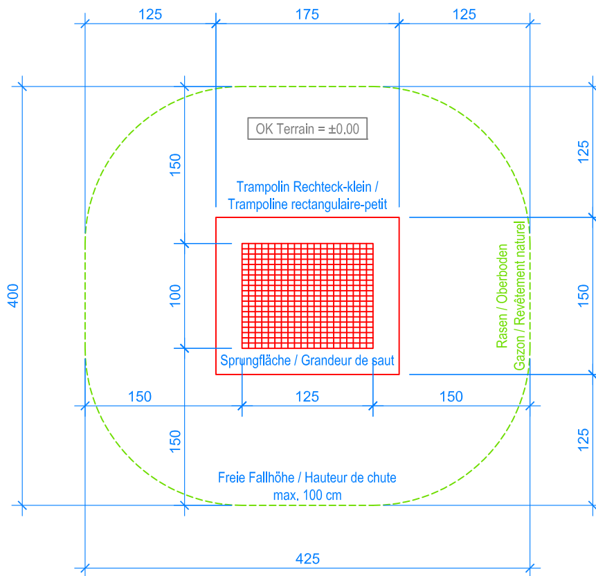
GRUNDRISS / PLAN 1:50
