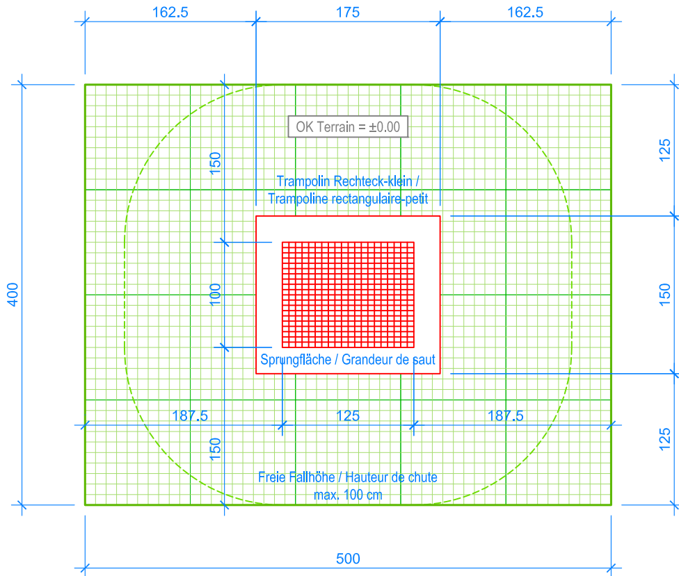
GRUNDRISS / PLAN 1:50
