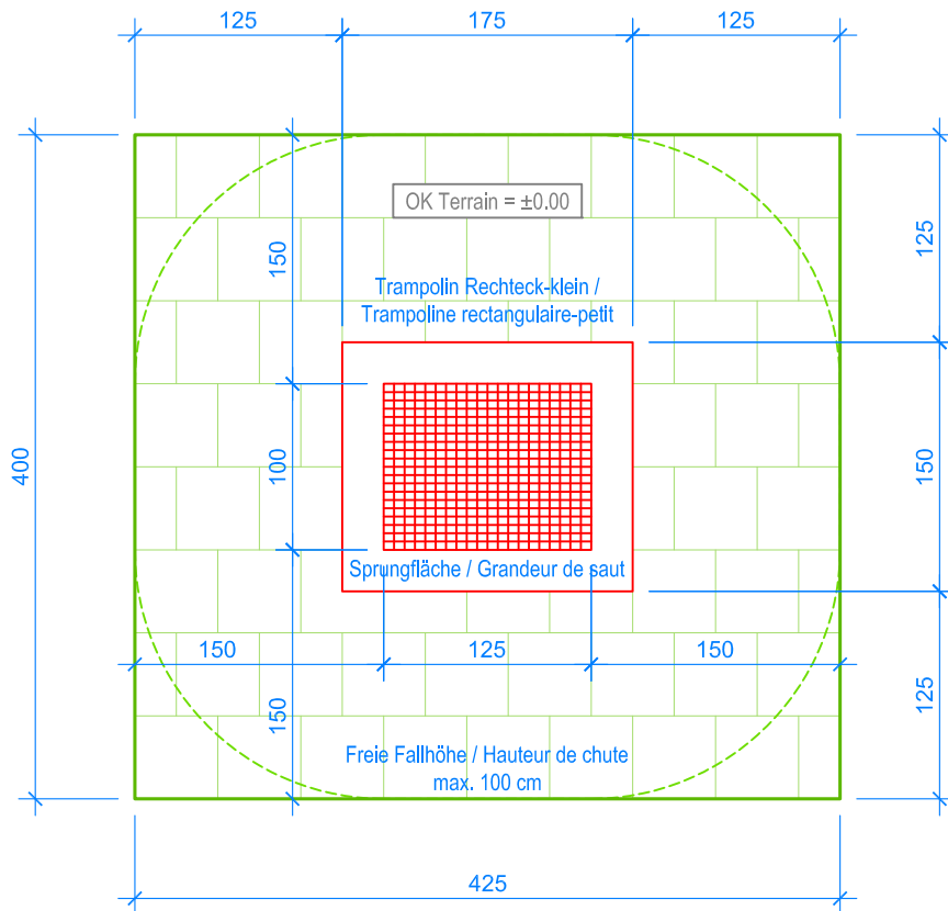
GRUNDRISS / PLAN 1:50
