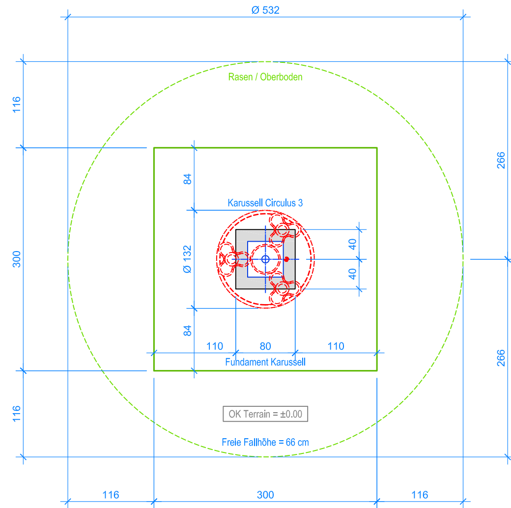
GRUNDRISS 1:50
