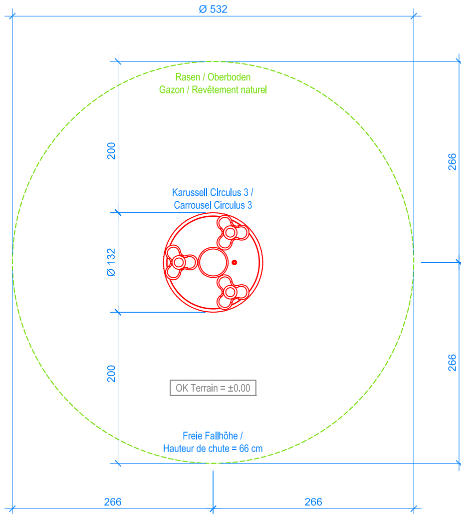
GRUNDRISS / PLAN 1:50
