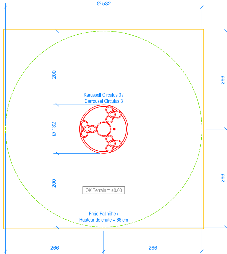
GRUNDRISS / PLAN 1:50
