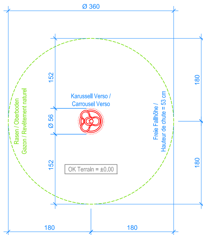
GRUNDRISS / PLAN 1:50
