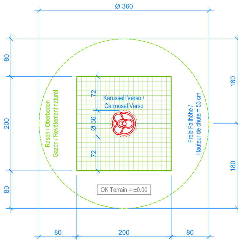
GRUNDRISS / PLAN 1:50
