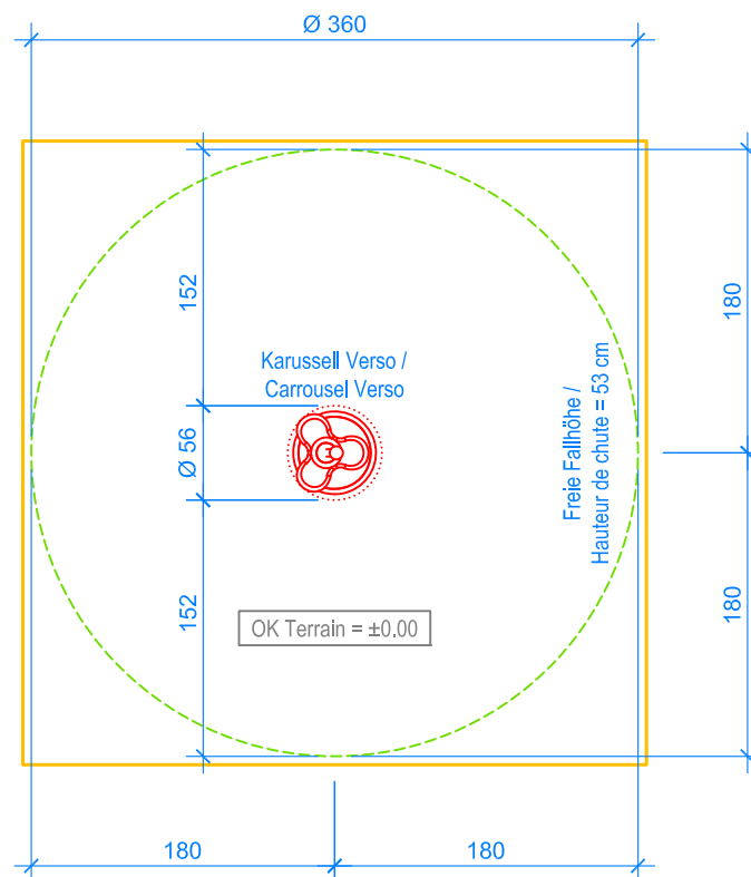
GRUNDRISS / PLAN 1:50
