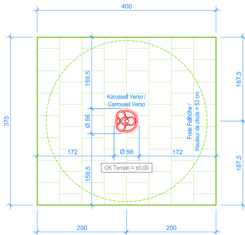
GRUNDRISS / PLAN 1:50
