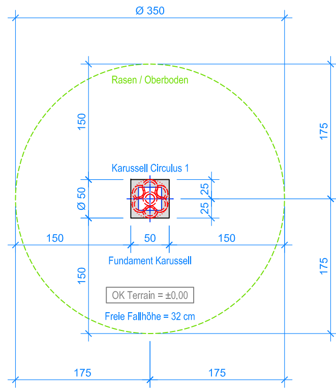
GRUNDRISS 1:50
