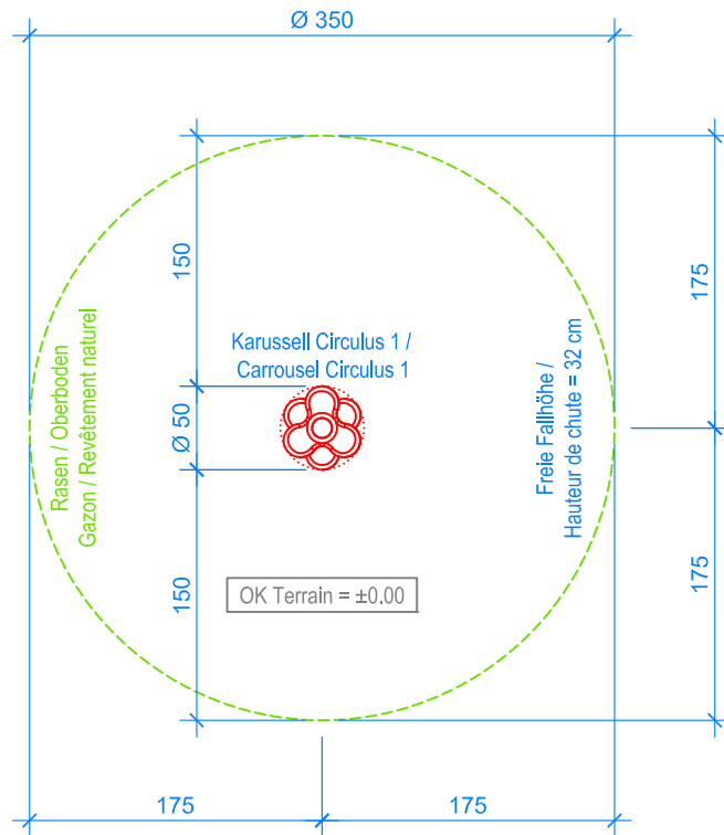
GRUNDRISS / PLAN 1:50
