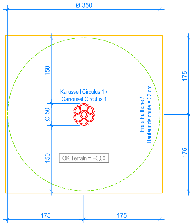
GRUNDRISS / PLAN 1:50
