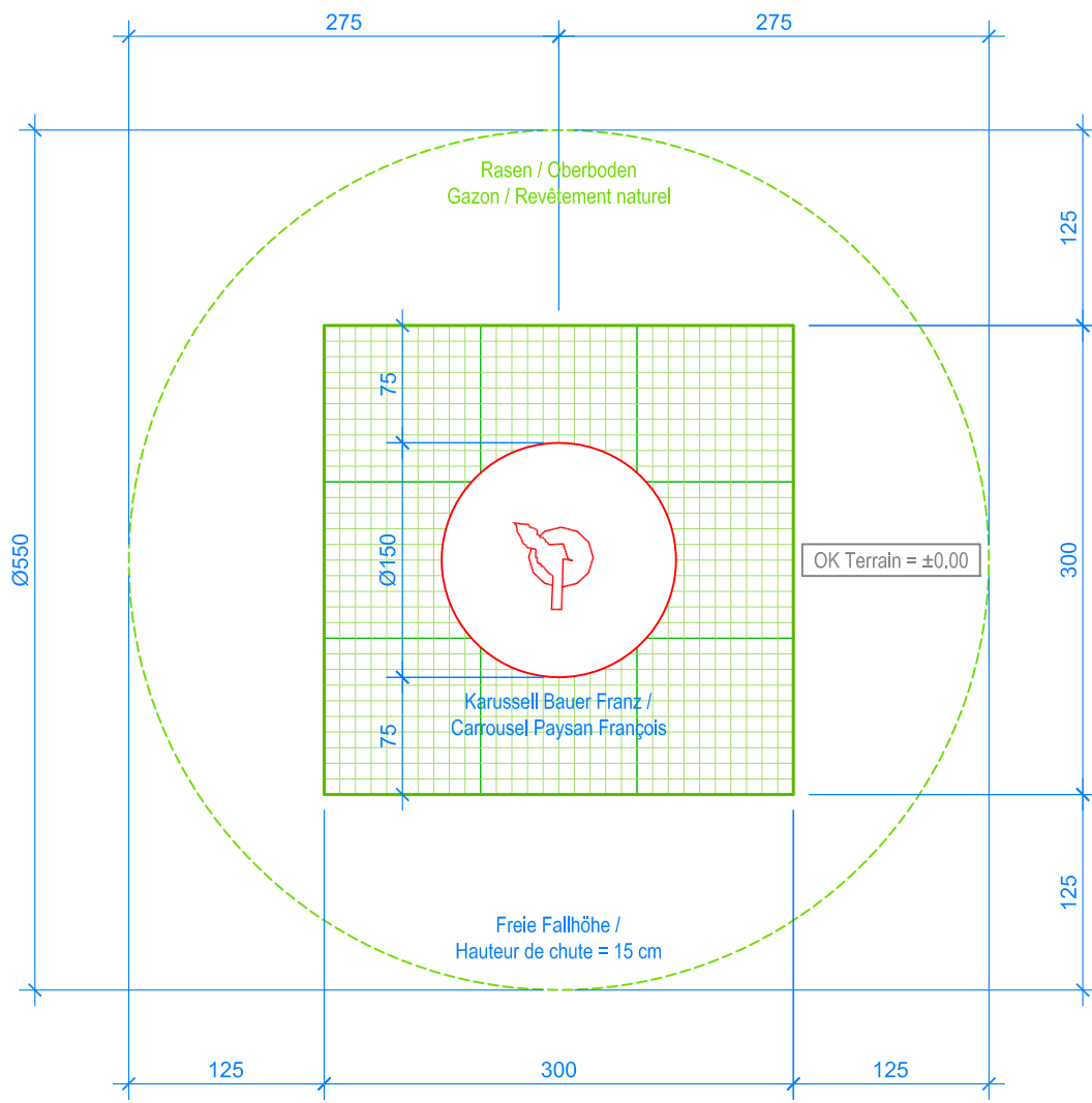
GRUNDRISS / PLAN 1:50
