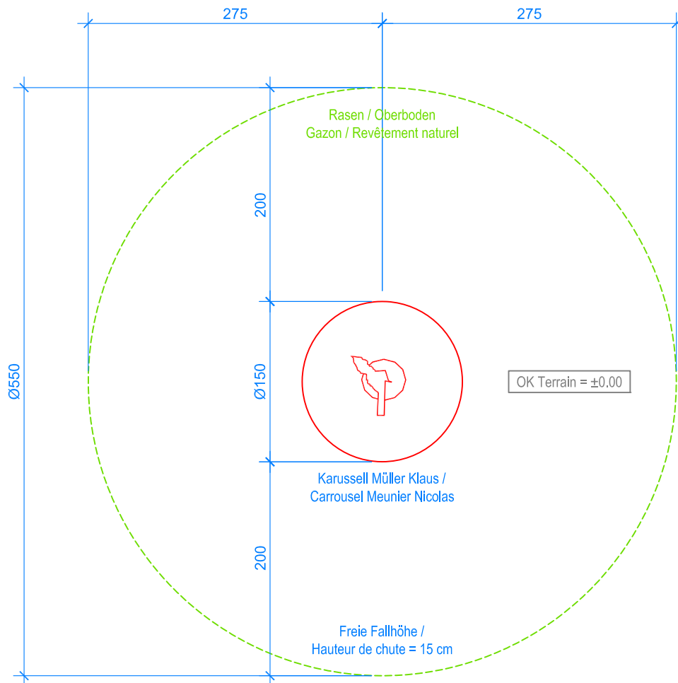
GRUNDRISS / PLAN 1:50
