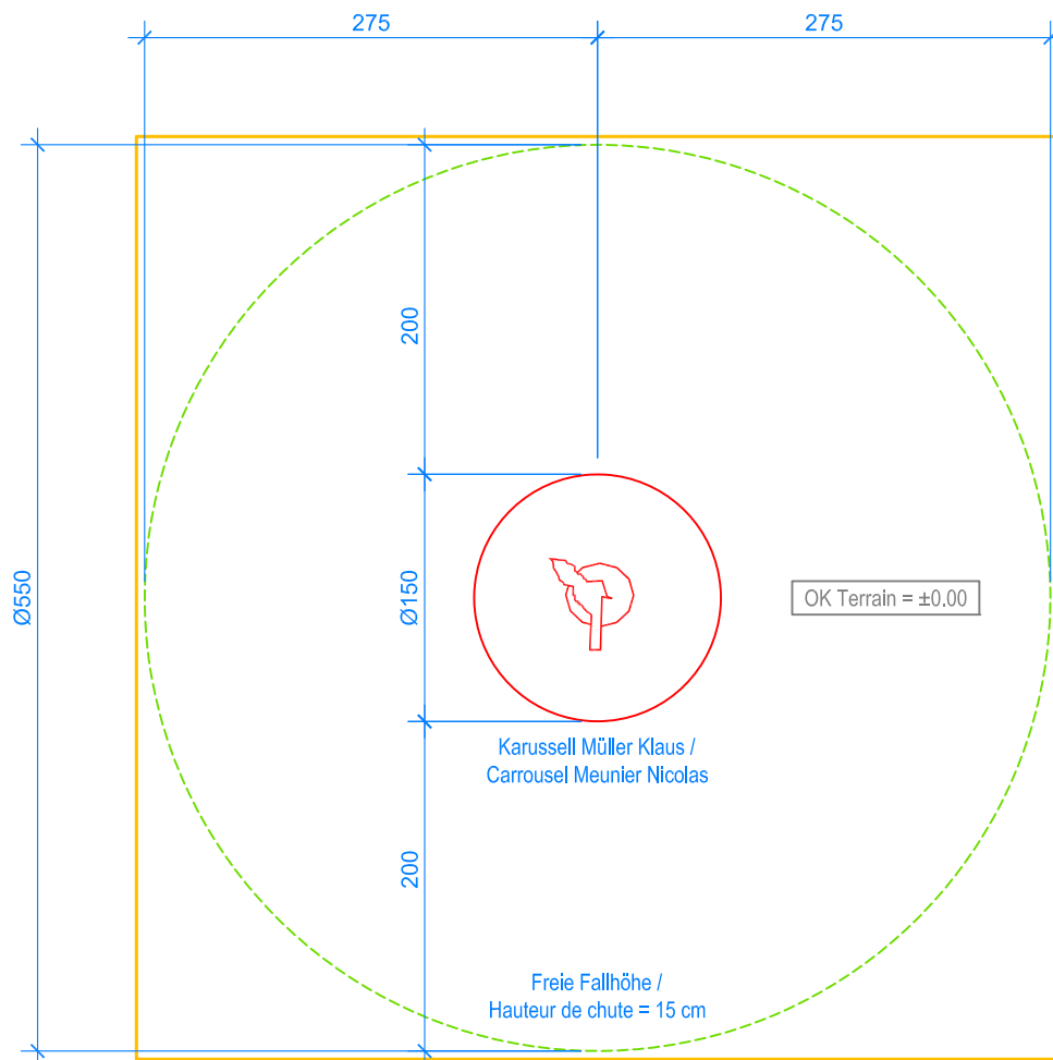
GRUNDRISS / PLAN 1:50
