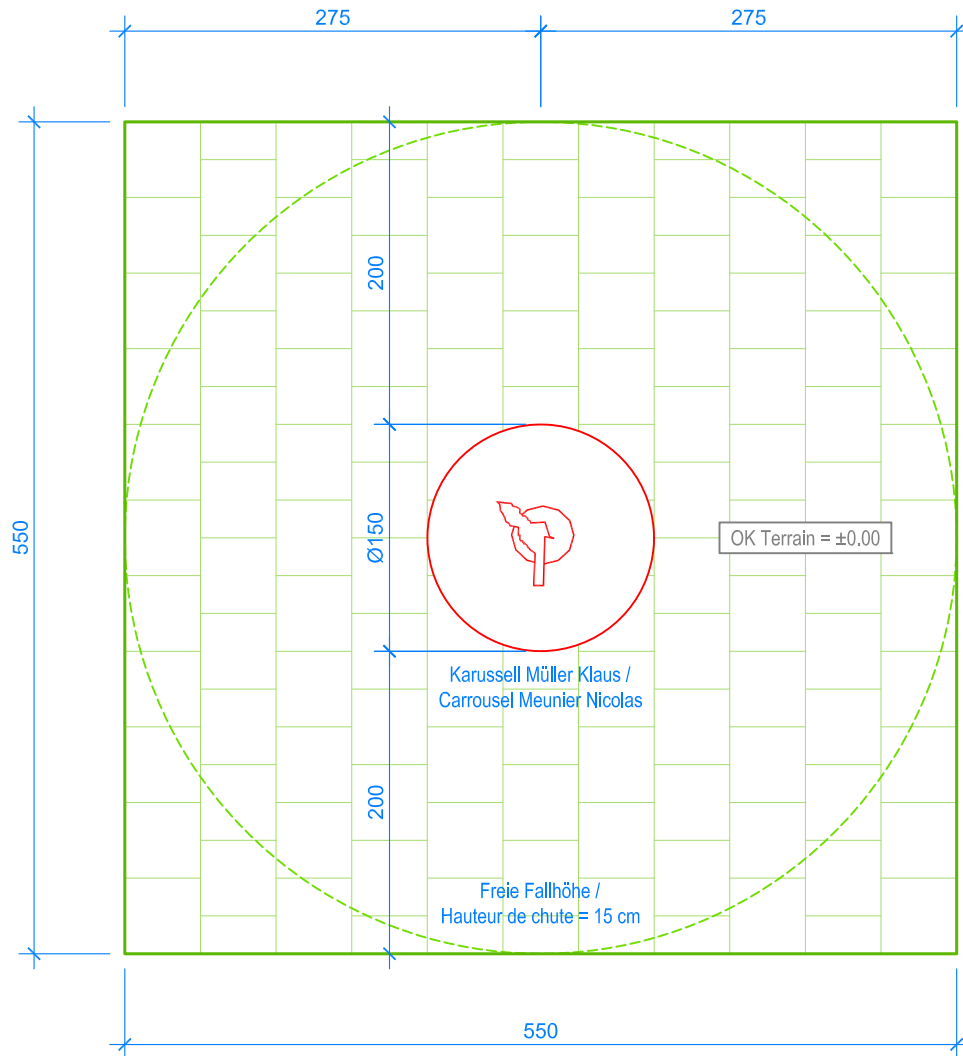
GRUNDRISS / PLAN 1:50
