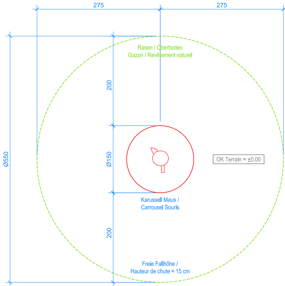
GRUNDRISS / PLAN 1:50
