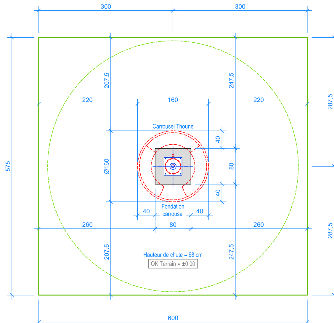
PLAN 1:50
