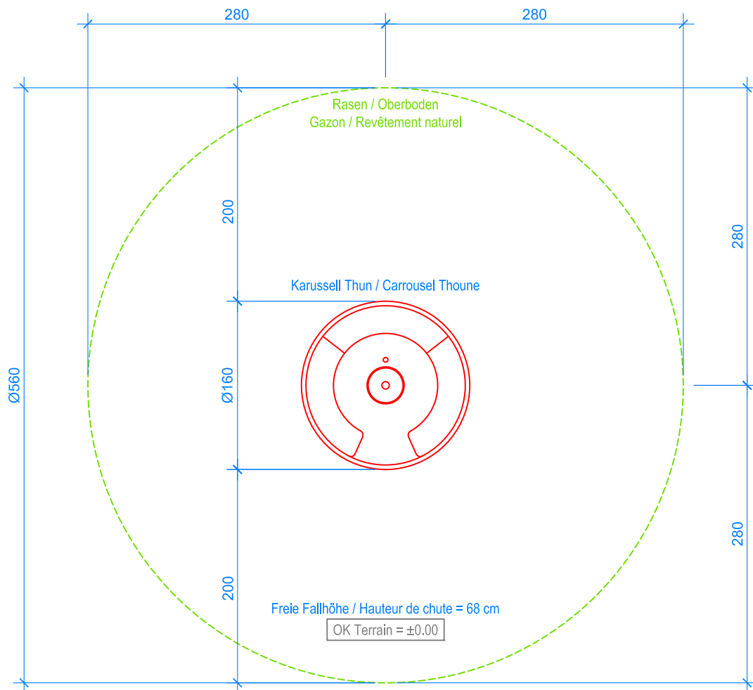
GRUNDRISS / PLAN 1:50
