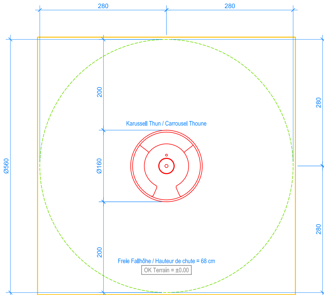
GRUNDRISS / PLAN 1:50
