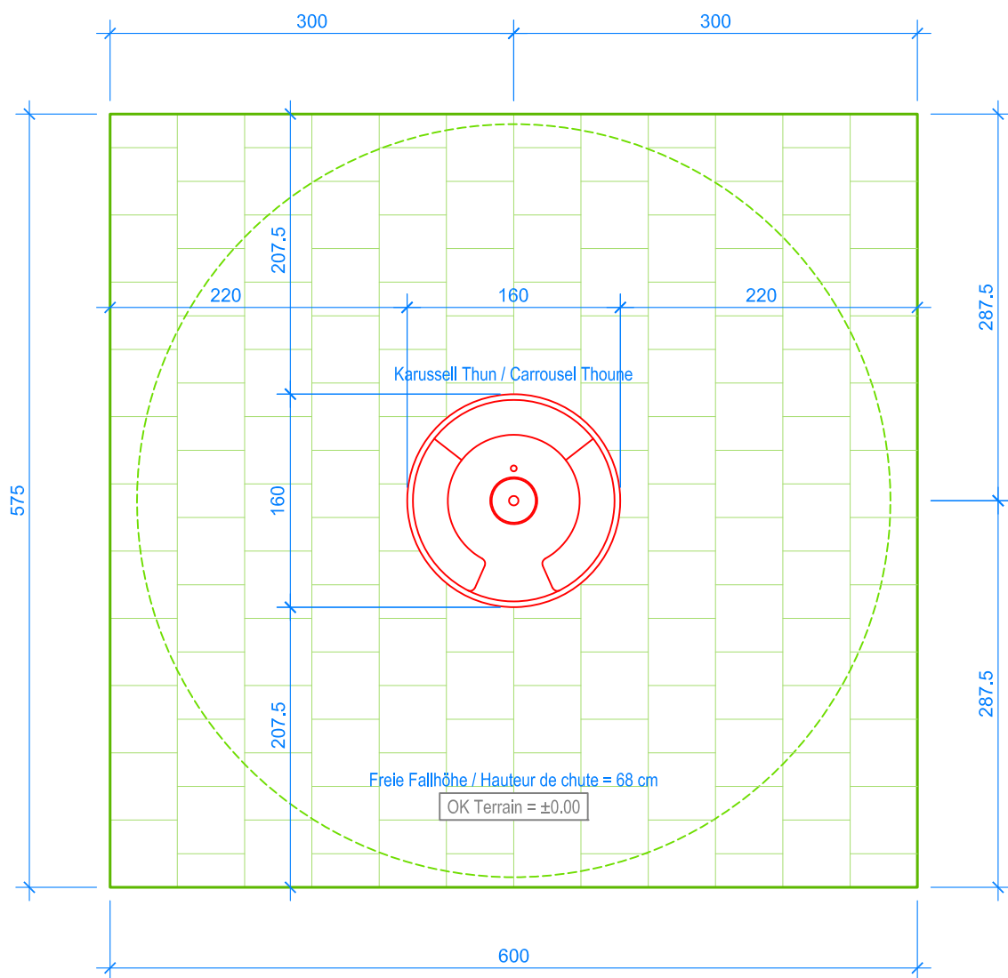
GRUNDRISS / PLAN 1:50
