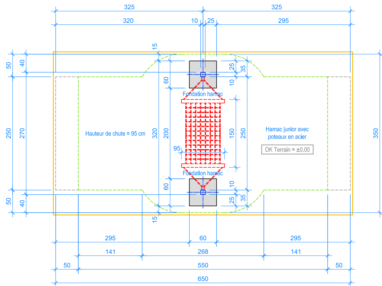
PLAN 1:50
