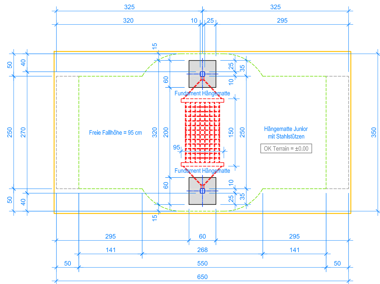
GRUNDRISS 1:50
