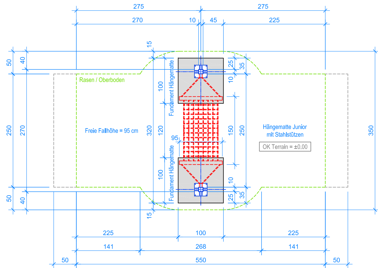
GRUNDRISS 1:50
