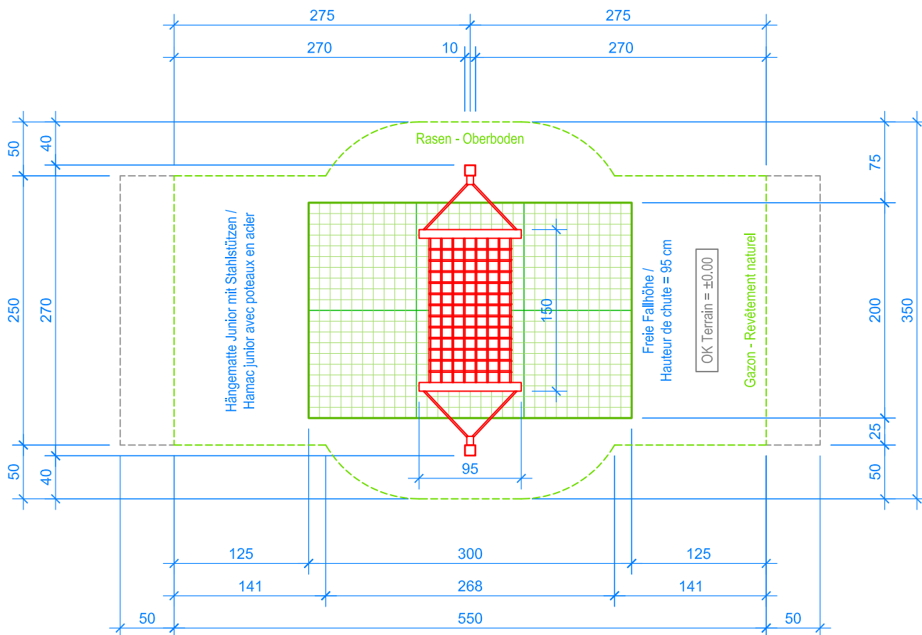
GRUNDRISS / PLAN 1:50
