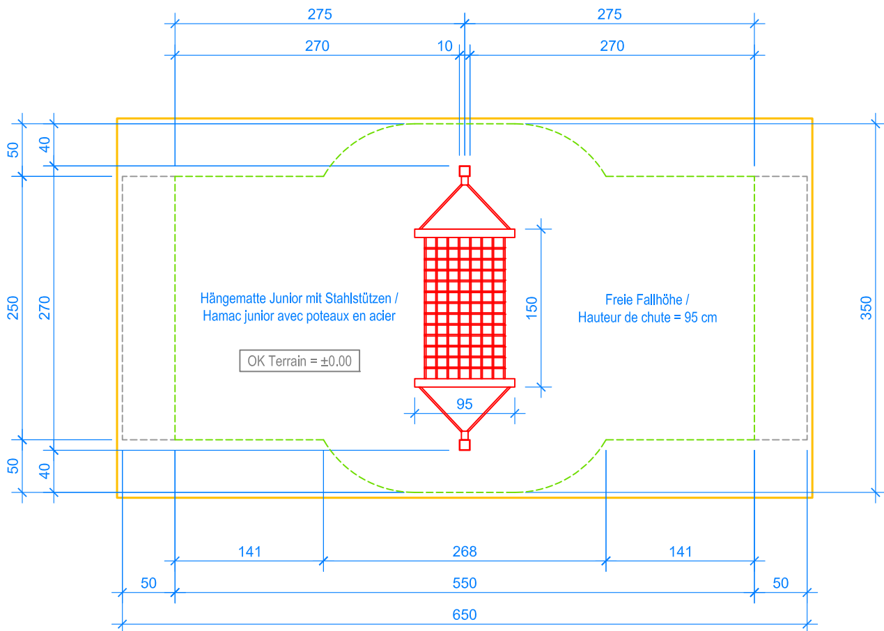
GRUNDRISS / PLAN 1:50
