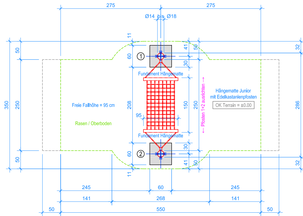
GRUNDRISS 1:50
