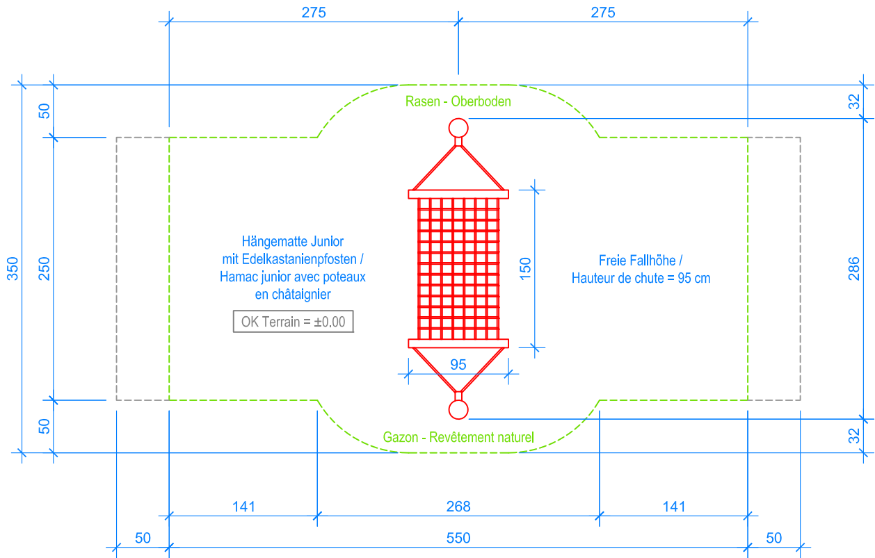
GRUNDRISS / PLAN 1:50
