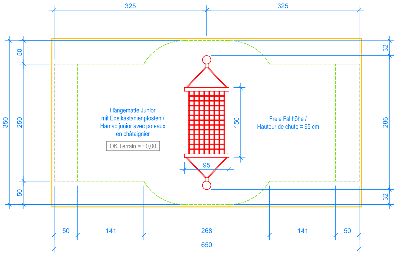
GRUNDRISS / PLAN 1:50
